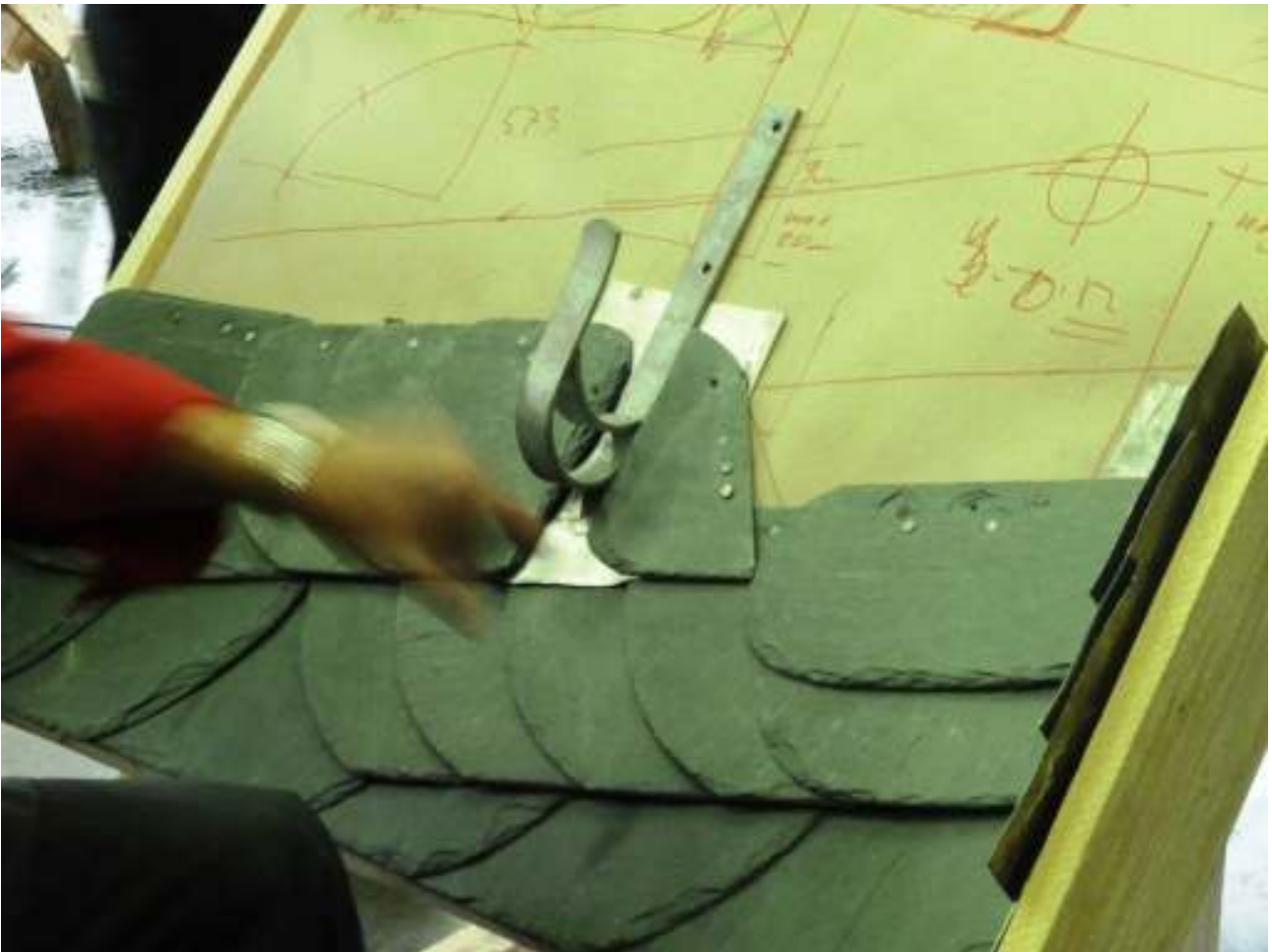
Dachhaken-Einbau in der Altdeutschen Schieferdeckung
